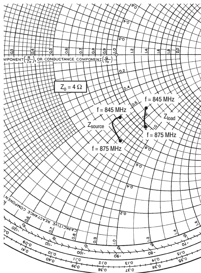
MRF374A
