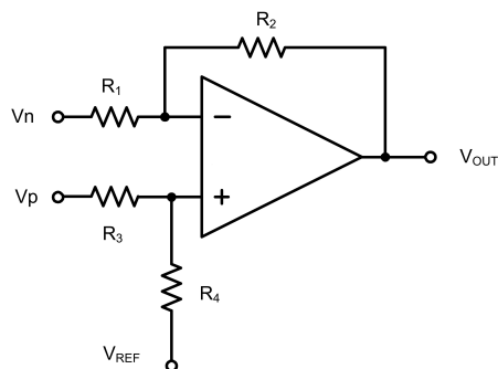
差分放大器
