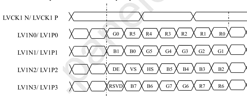
Fig. 5.4 VESA format
