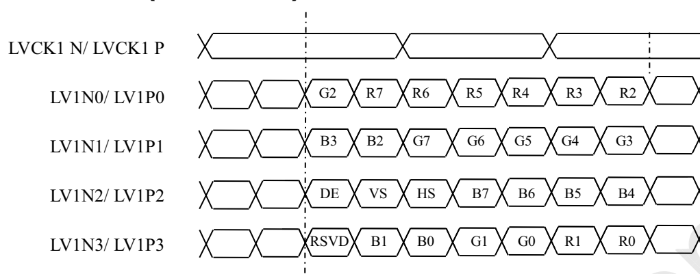
Fig. 5.5 JEIDA format
