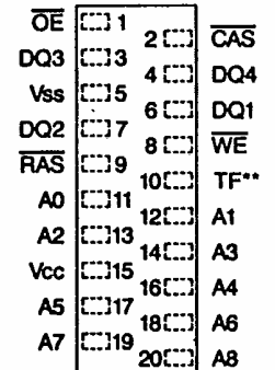
MT4C4256E 20 Pin ZIP
