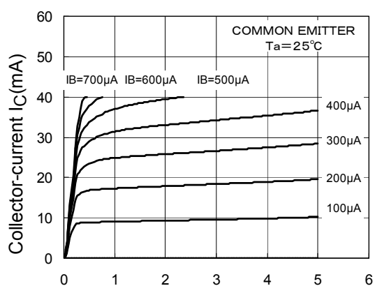
I_C-V_{CE}
