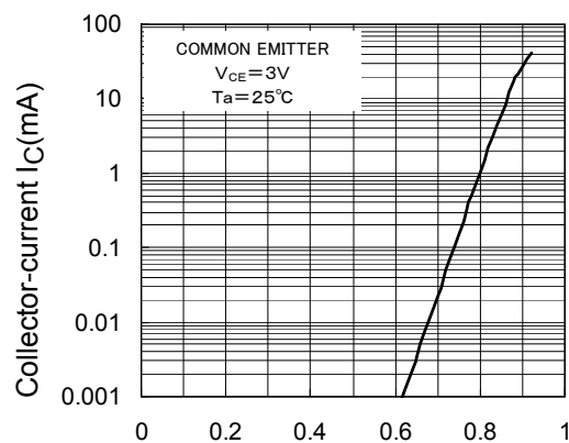
I_C-V_{BE}
