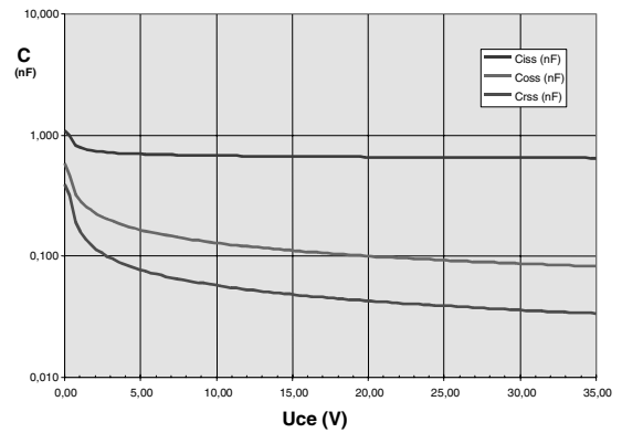
Typ. capacitances
