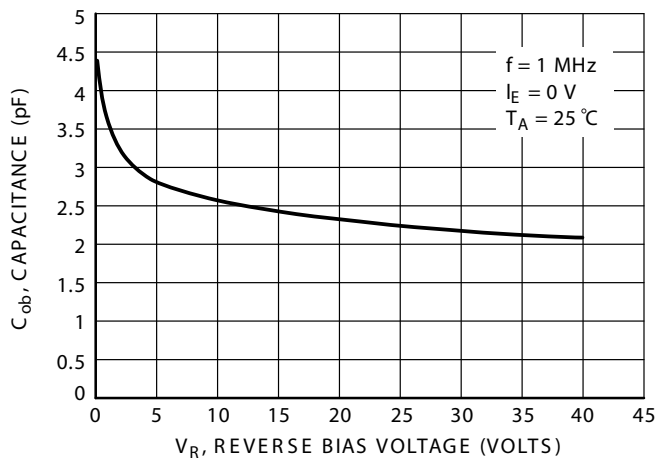
FIG24. Output Capacitance
