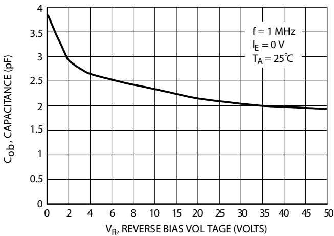
FIG19. Output Capacitance
