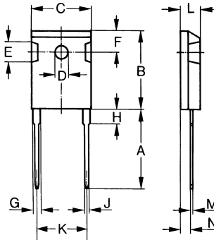
Dimensions TO-247AC
