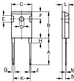
Dimensions TO-247AC
