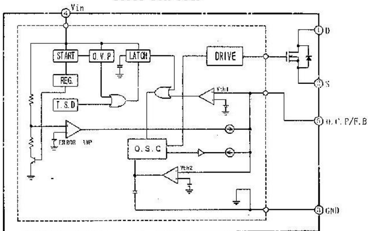
IC901 STR-5643
