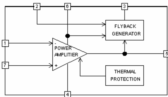
IC601 STV9302A
