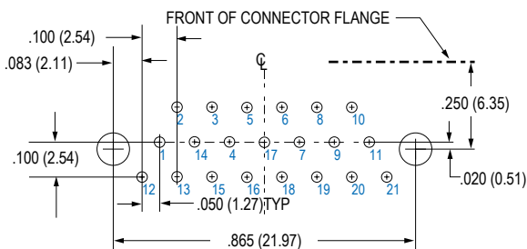
21 PIN MWDM-21PCBR
