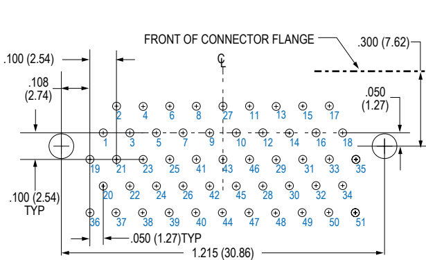
51 PIN MWDM-51PCBR
