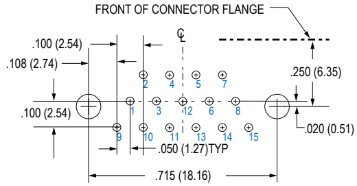
15 PIN MWDM-15PCBR
