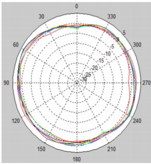
5.8G horizontal pattern
