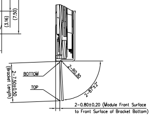
SECTION YY-YY SCALE 5:1
