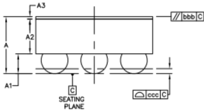
NAU8315/NAU83U15 9 Ball WLCSP Package
