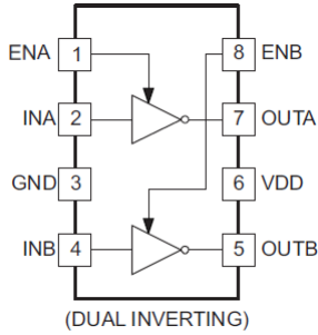
NCP81071A
