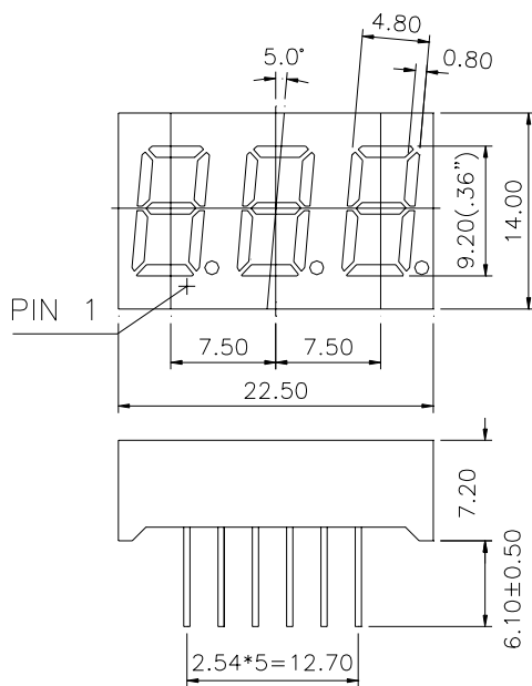
NET-3631AS
