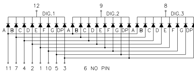
NET-3631AS
