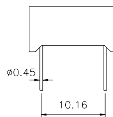
NET-3632AS
