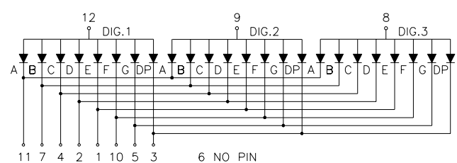
NET-3632AS
