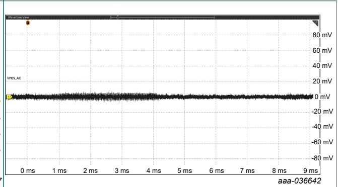
Fig. 24. V_{POS} output ripple ( I_{POS} = 0 mA)
