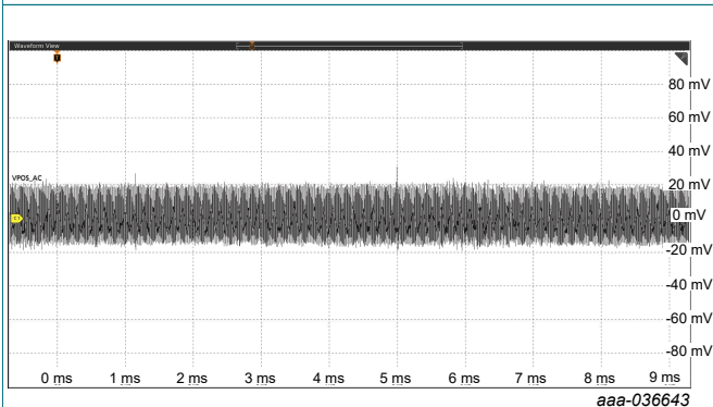
Fig. 25. V_{POS} output ripple ( I_{POS} = 40 mA)
