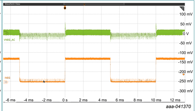
Fig. 36. Load transient
