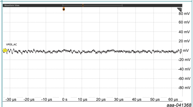
Fig. 26. V_{POS} output ripple ( I_{POS} = 120 mA)
