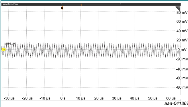
Fig. 23. V_{NEG} output ripple ( I_{NEG} = 120 mA)
