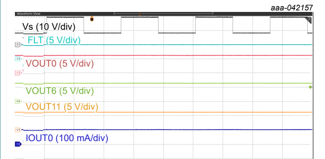
Fig. 19. Vs transient
