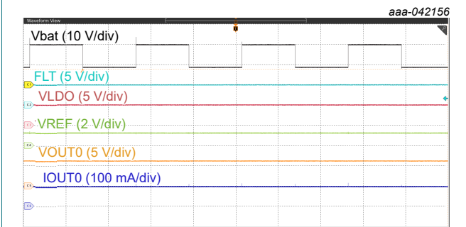
Fig. 18. Vbat transient
