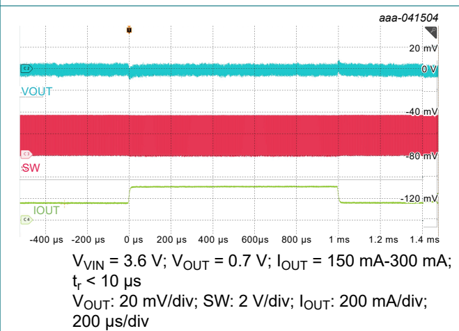
Fig. 36. Load transient
