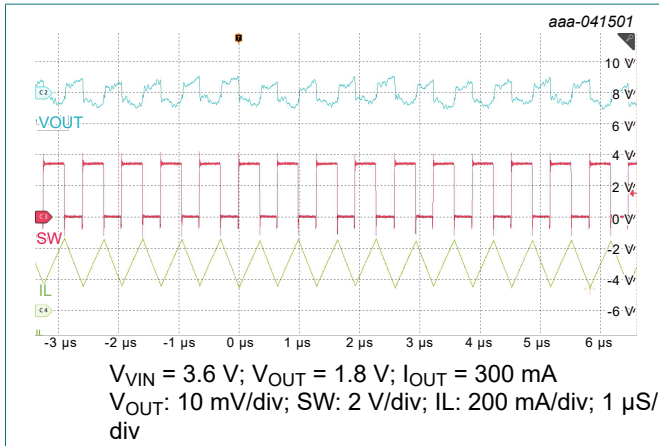
Fig. 33. Output ripple
