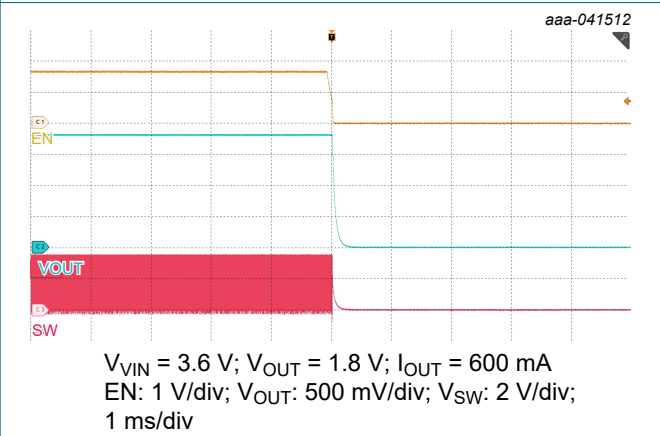
Fig. 44. EN OFF
