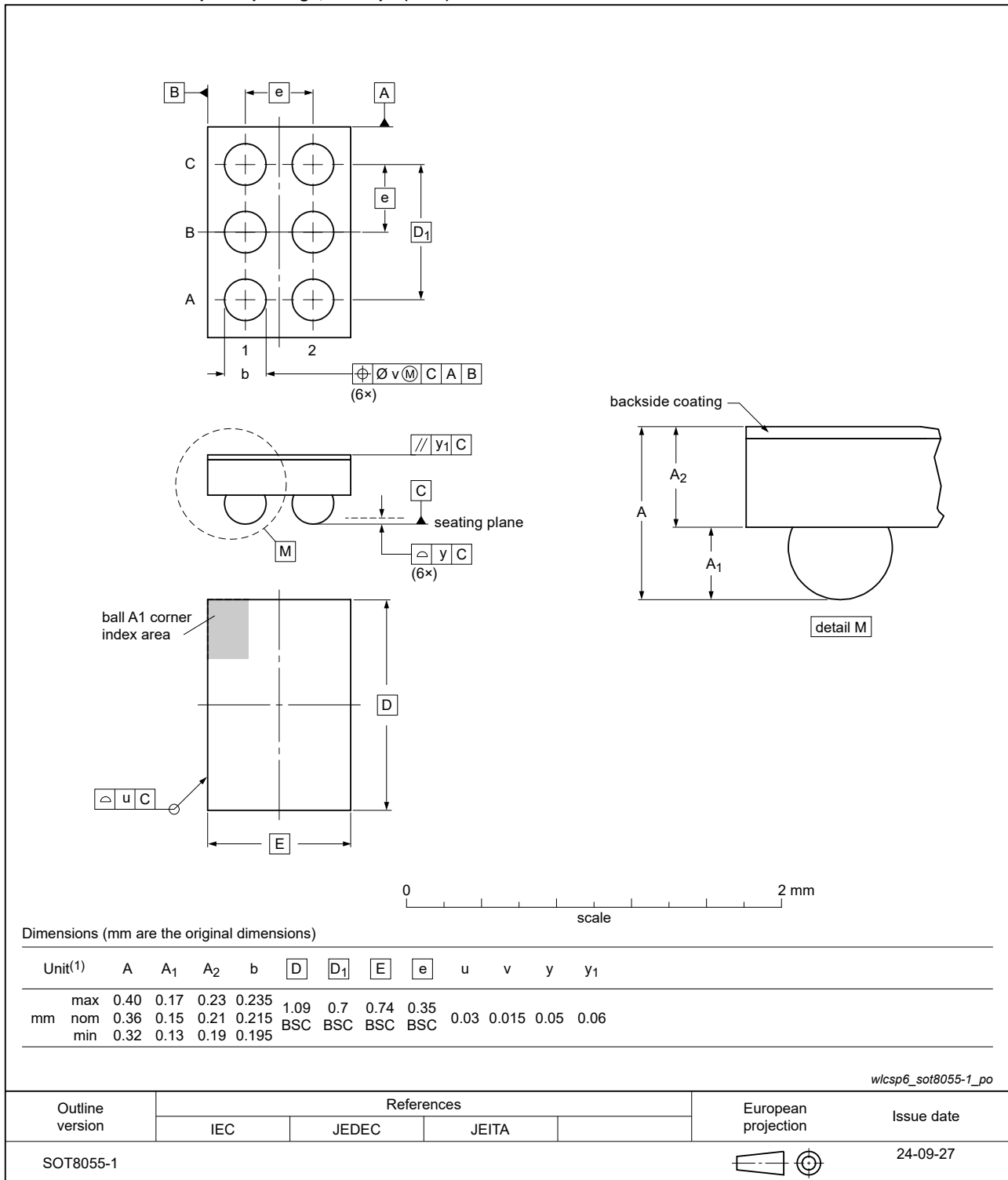
Fig. 47. Package outline SOT8055-1 (WLCSP6)
