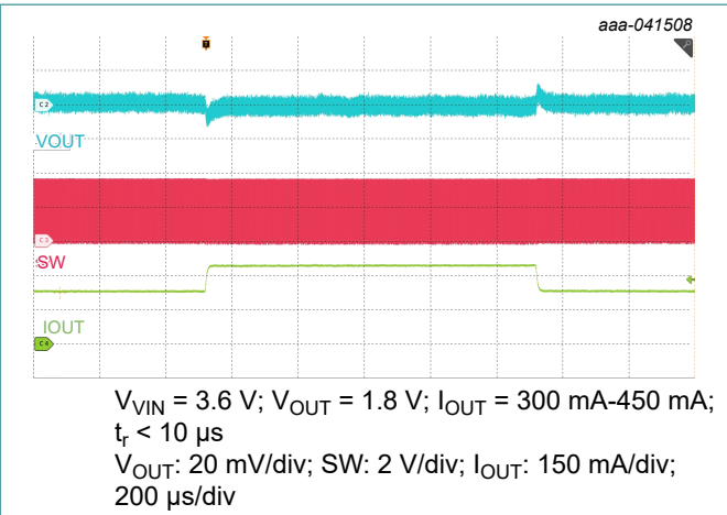
Fig. 40. Load transient
