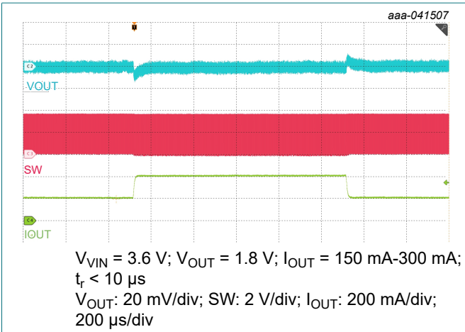
Fig. 39. Load transient
