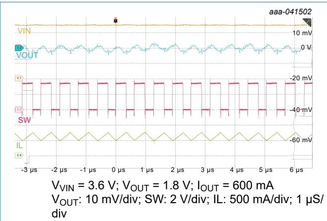
Fig. 34. Output ripple
