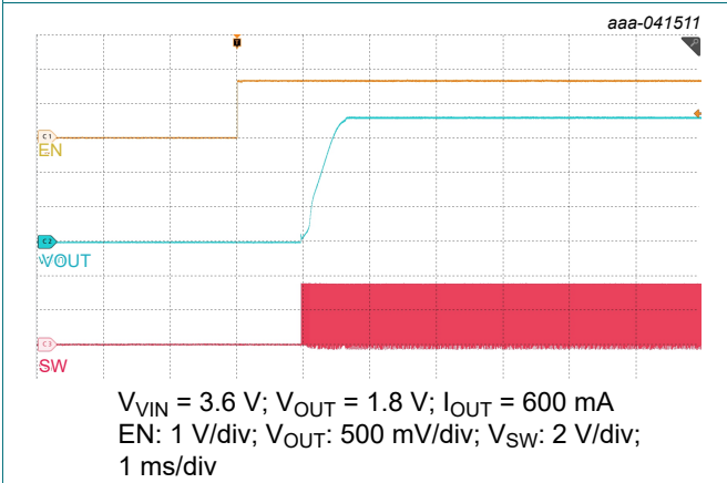
Fig. 43. EN startup
