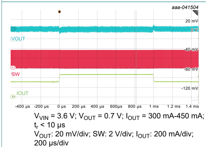
Fig. 37. Load transient
