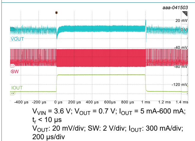
Fig. 35. Load transient
