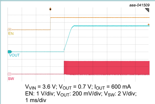
Fig. 41. EN startup
