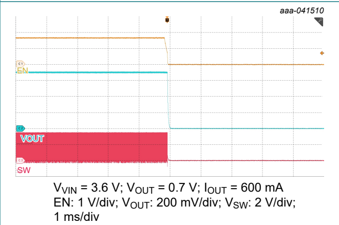
Fig. 42. EN OFF
