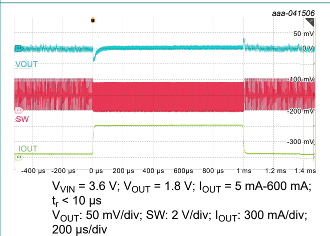
Fig. 38. Load transient
