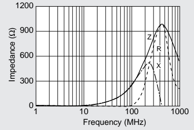
BLM10B102SD
