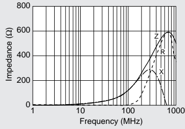
BLM10B601SD
