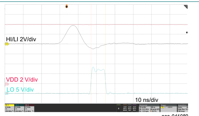
Fig. 24. Minimum turn-on time
