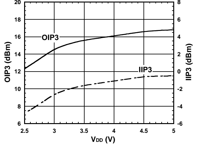
OIP3, IIP3 vs. V DD
