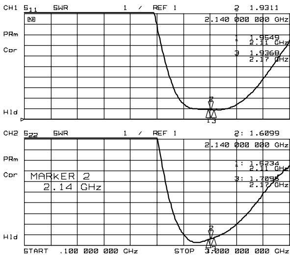
VSWR
