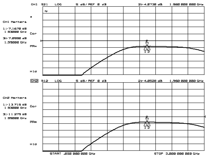
S21, S12
