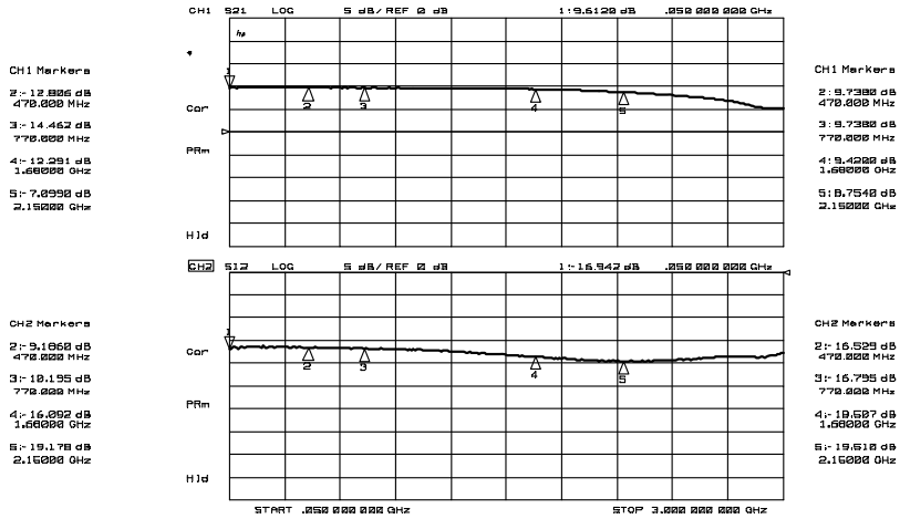
S21, S12
