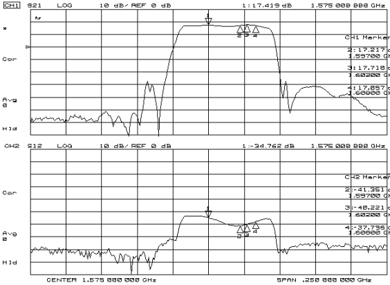
S21, S12
