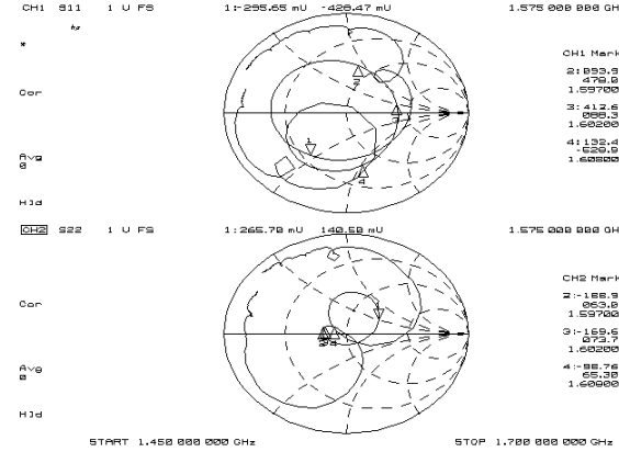
Zin, Zout
