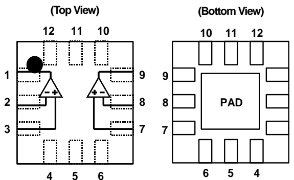
NJM2904CME2 (Note1, 2, 3)
