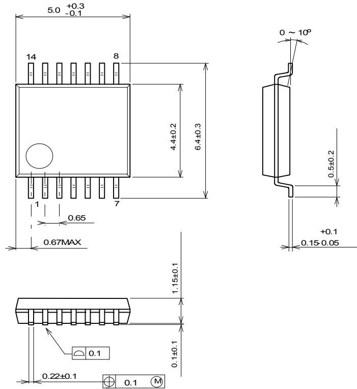
SSOP14 Package
