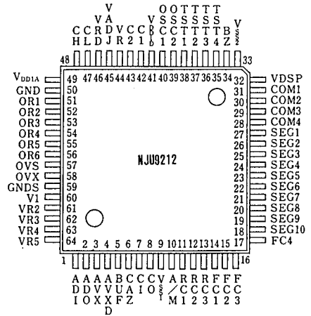
NJU9212F
