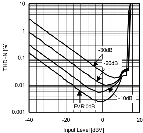
Volume THD+N vs. Input Level INPUT:LAIN OUTPUT:L.OUT f=1kHz V+=7V V-=-7V BW=10Hz-80kHz Ta=25°C
