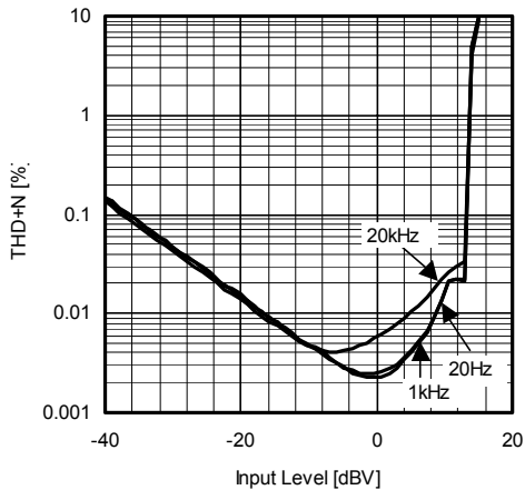
Volume THD+N vs. Input Level INPUT:LAIN OUTPUT:L.OUT V+=7V V-=-7V RL=10kΩ 0dB setting BW=10Hz-80kHz Ta=25°C
