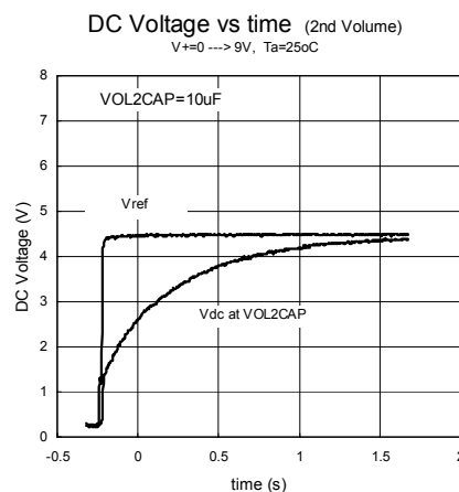
Fig.6-4.VOL2CAP=10uF
