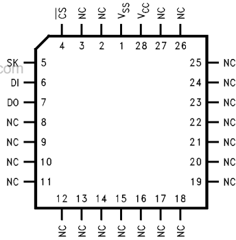
NM29A040V NS Package Number V28A
