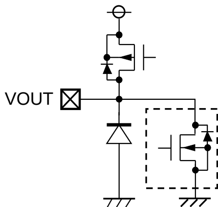
VOUT pin
