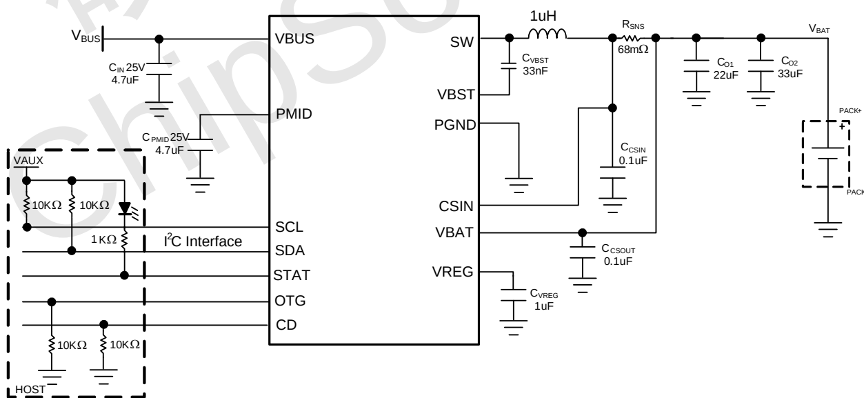
图 1 NS2157 典型应用电路
