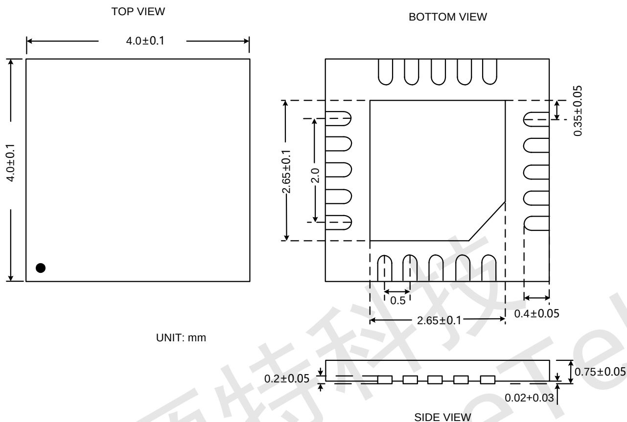
图 29 NS2157 QFN 封装信息
