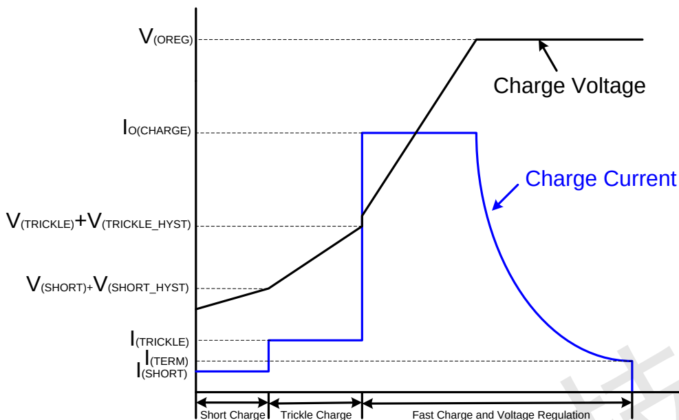
图 14 NS2157 Without Input Current Limit 充电流程图
