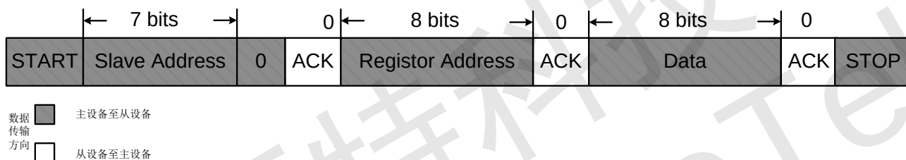
图 22 I 2 C 写操作
