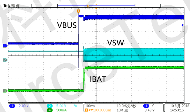
图 6 V_{\text{BUS}}=0-5\text{V} , I_{\text{IN\_LIMIT}}=0.9\text{A} , V_{\text{BAT}}=3.8\text{V} , Adapter Insertion
