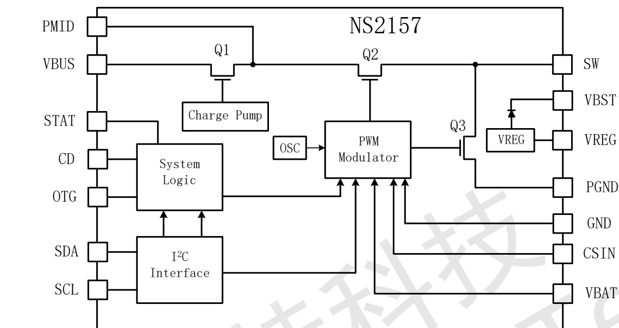
图 13 NS2157 功能结构框图
