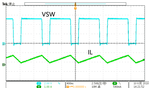
图 4 V_{\text{BUS}}=5.5\text{V} , V_{\text{BAT}}=3.8\text{V} , I_{\text{O(CHAARGE)}}=1.75\text{A} , PWM 充电波形
