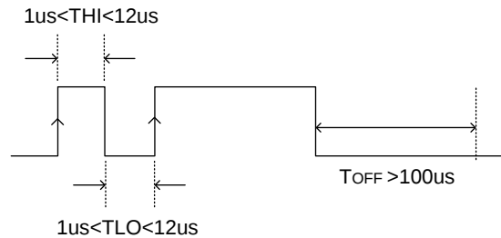
图5 一线脉冲时序图
