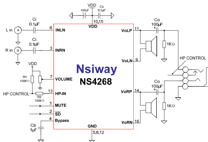
图1 NS4268 典型应用电路
