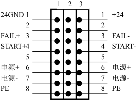
背视图
