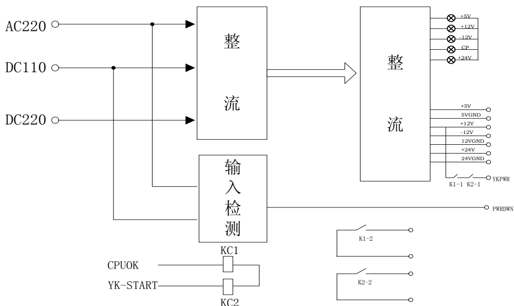
图 3.2 NSD200 系列通用测控装置电源模块原理框图
