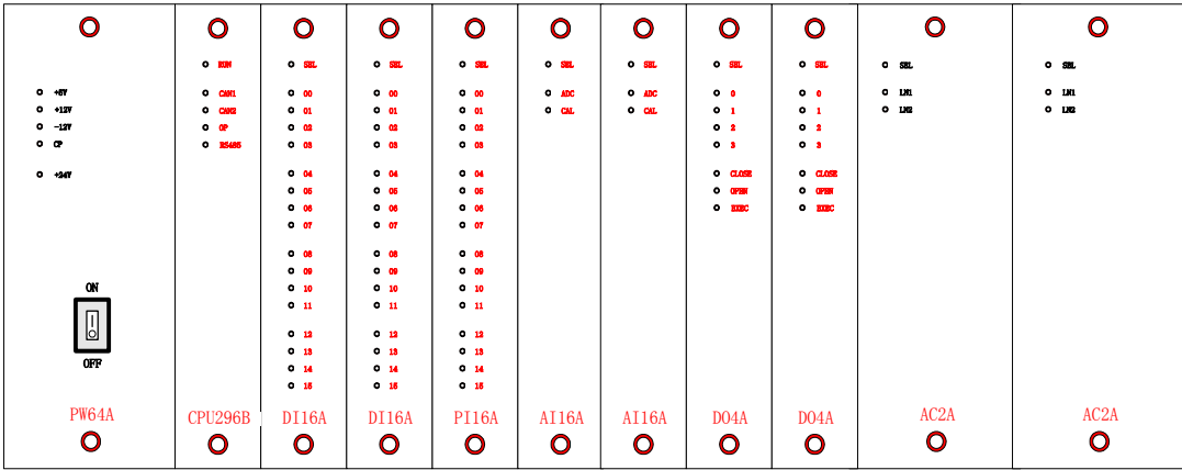
(a) 前视图
