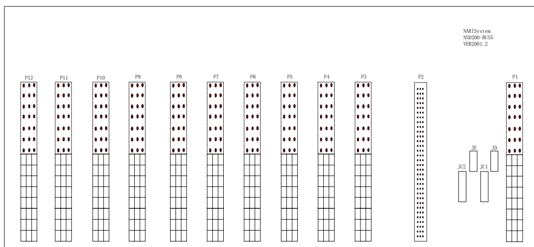
(b) 后视图
