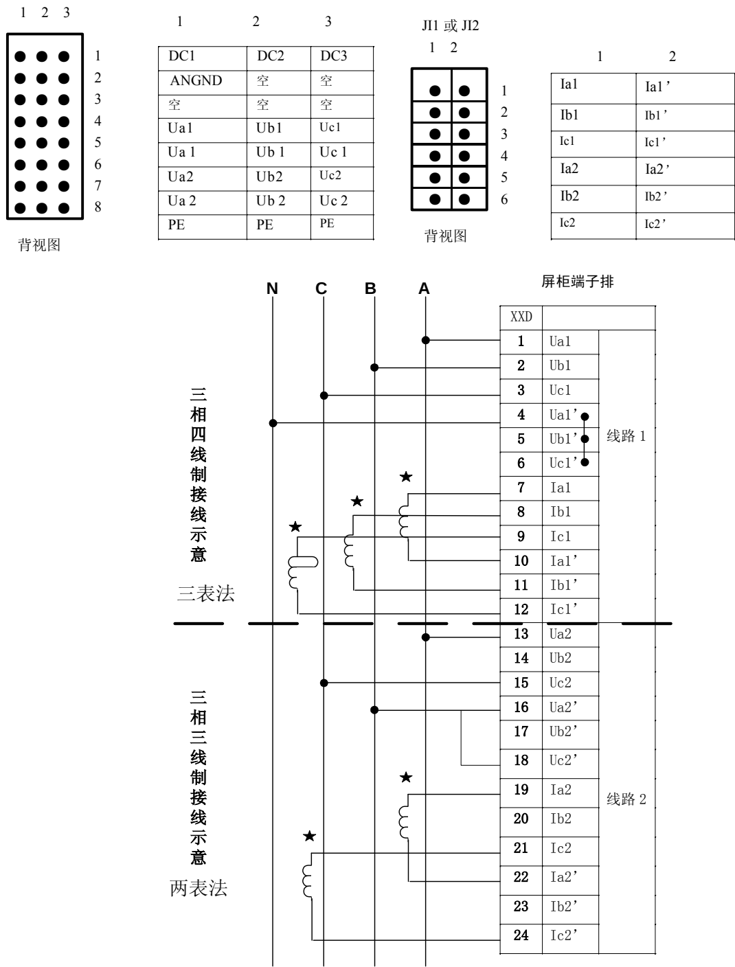
图 6.11 AC2A 模件端子定义
