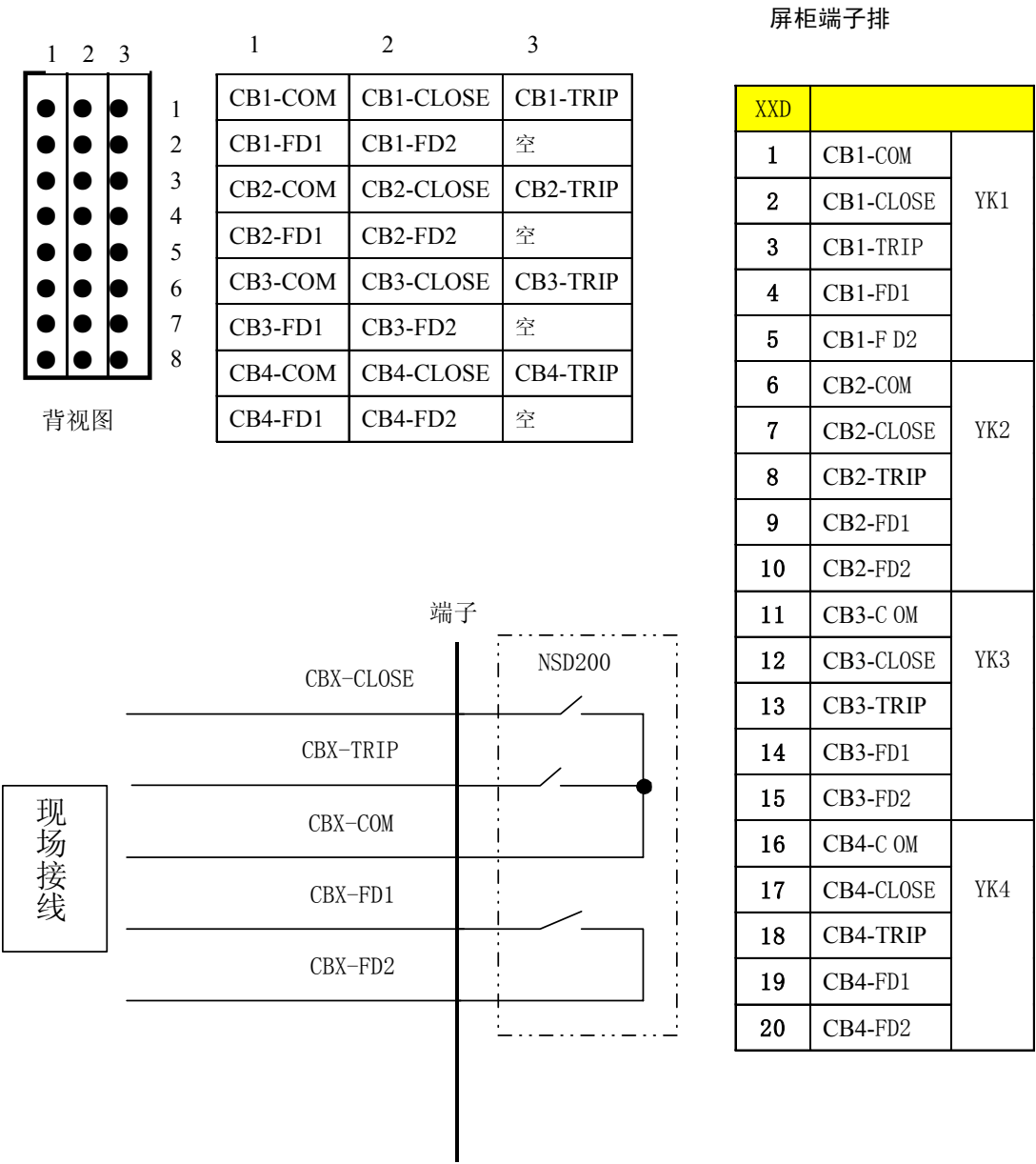
图 6.10 D04A 模件端子定义
