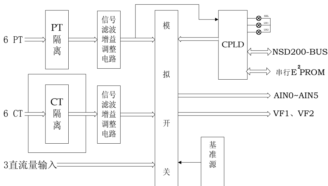
图 3.9 NSD200 系列通用测控装置 AC2A 模件原理框图
