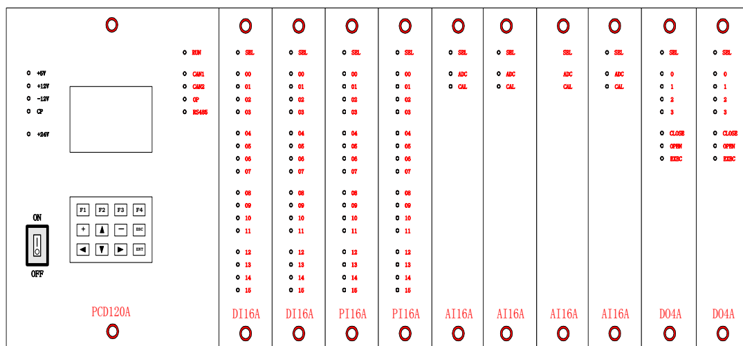
(a) 前视图
