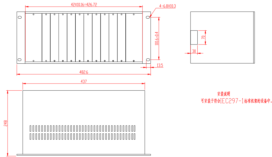
NSD200 系列测控装置尺寸图
