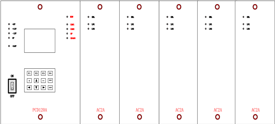
(a) 前视图
