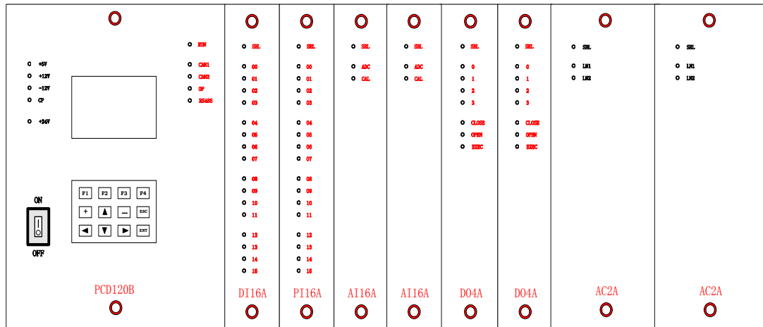
(a) 前视图
