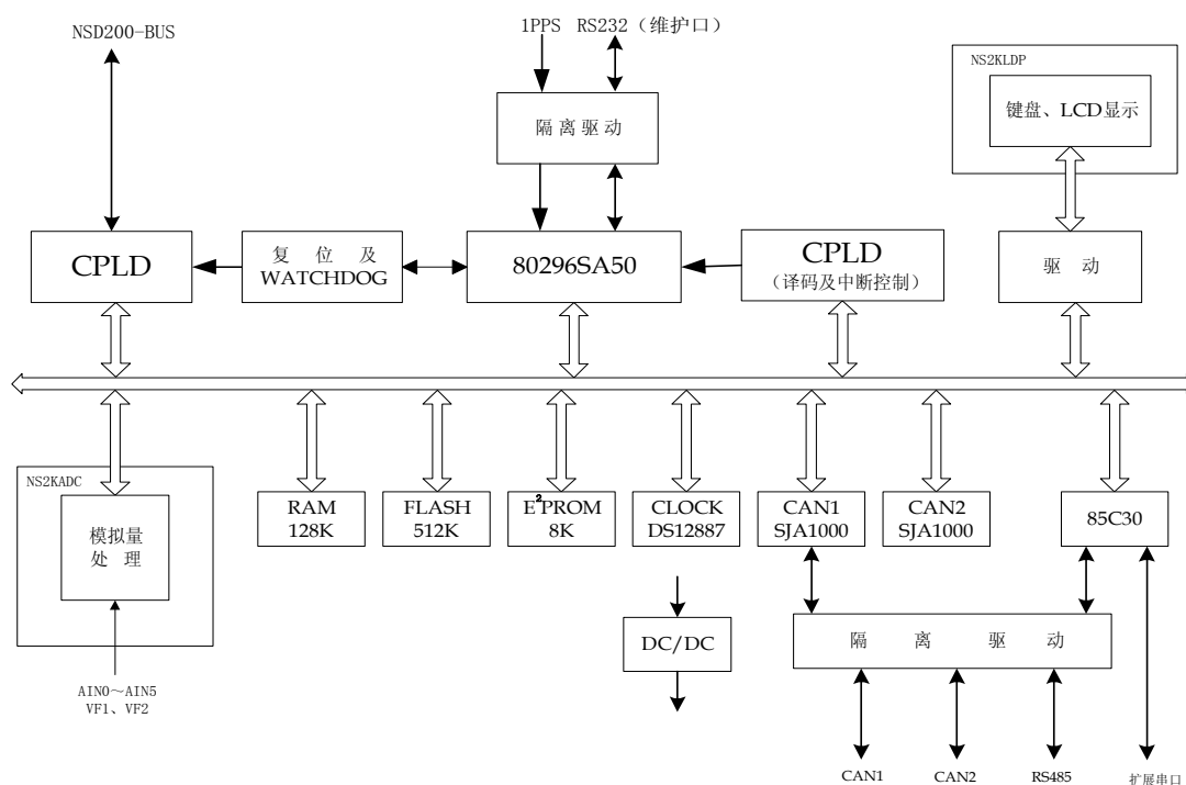
图 3.3 NSD200 系列通用测控装置 CPU 模块原理框图
