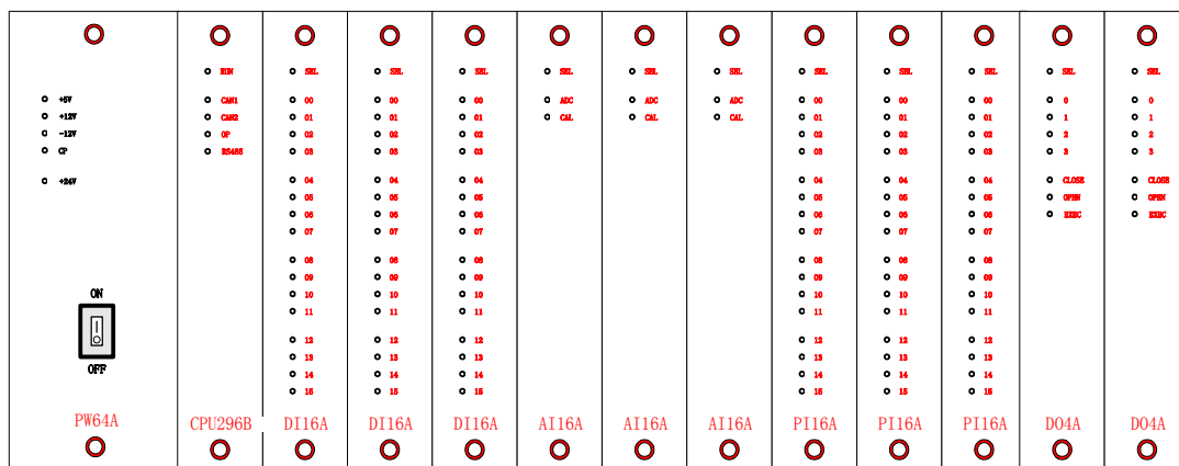
(a) 前视图
