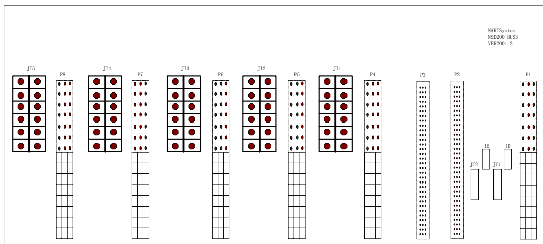
(b) 后视图
