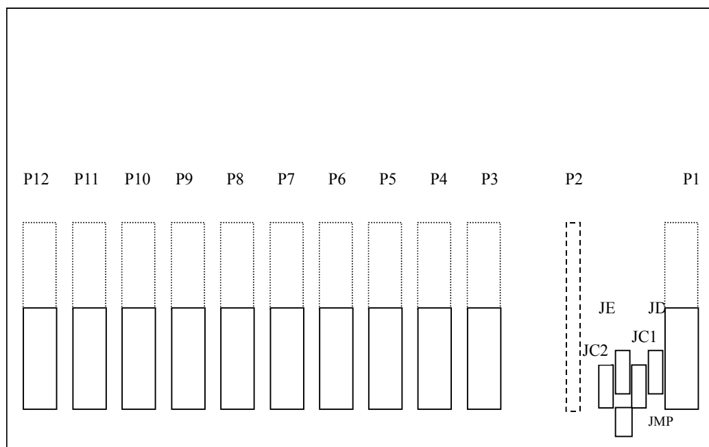
图 6.16 NSD205 背视图
