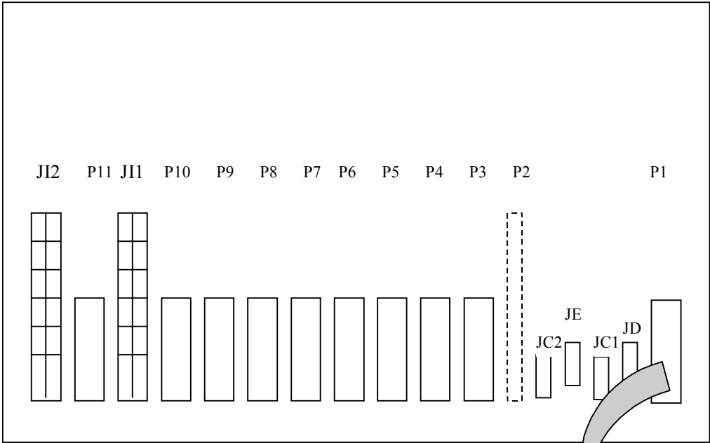
NSD200 背面示意图
