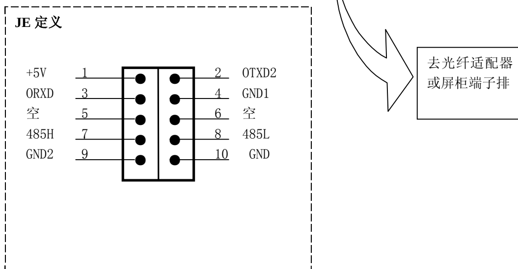
图 6.5 RS485 串口通讯接线图
