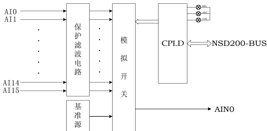
图 3.6 NSD200 系列通用测控装置 AI16 模件原理框图
