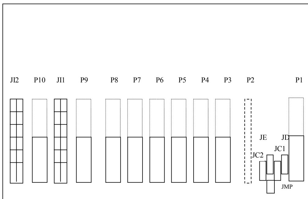
图 6.15 NSD204 背视图
