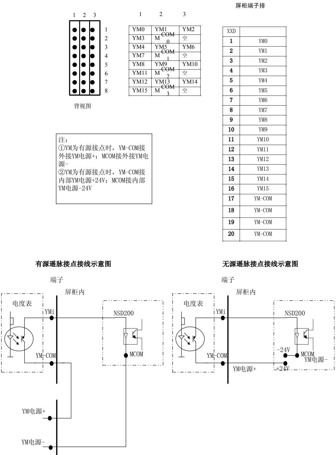
图 6.8 PI16A 模件端子定义
