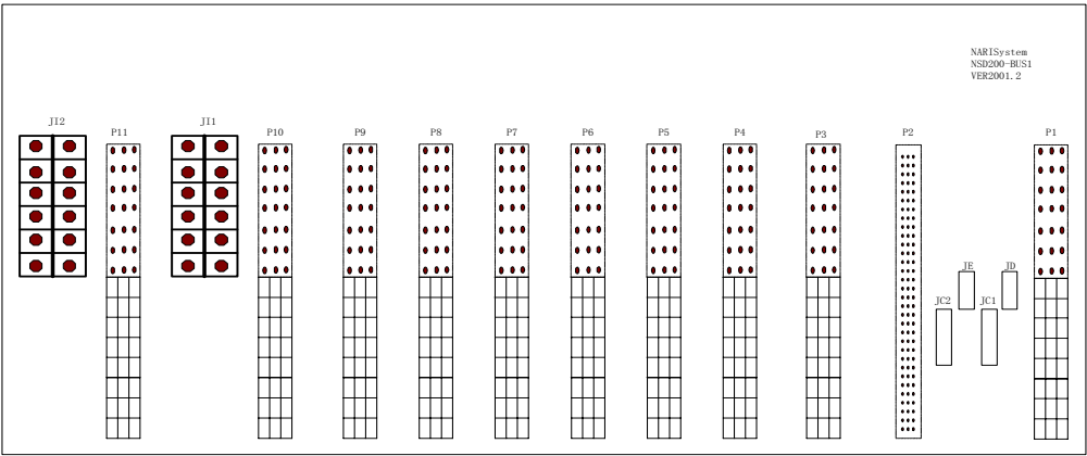
(b) 后视图
