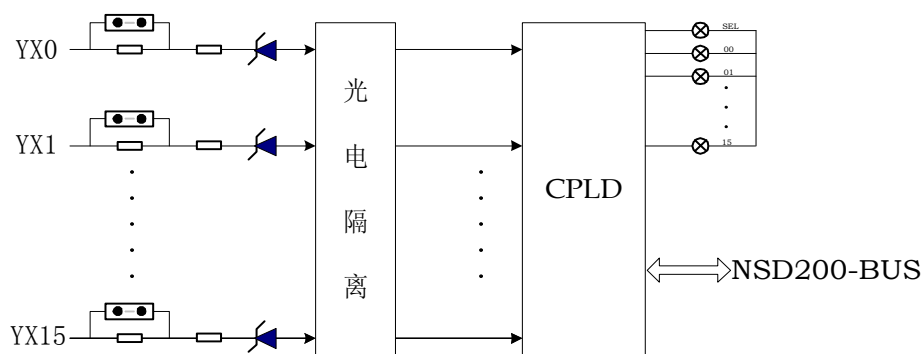
图 3.8 NSD200 系列通用测控装置 DI16A 模件原理框图
