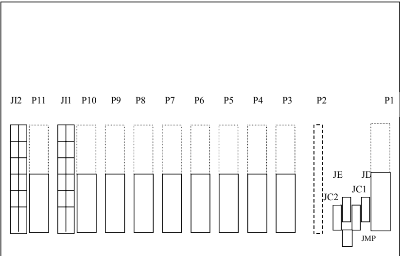
图 6.12 NSD201 背视图
