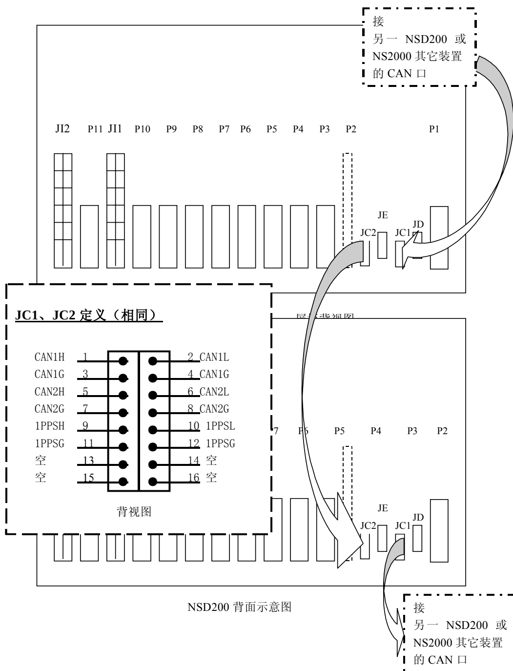
图 6.3 CAN 通讯接线图
