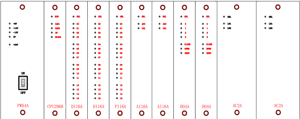
(a) 前视图
