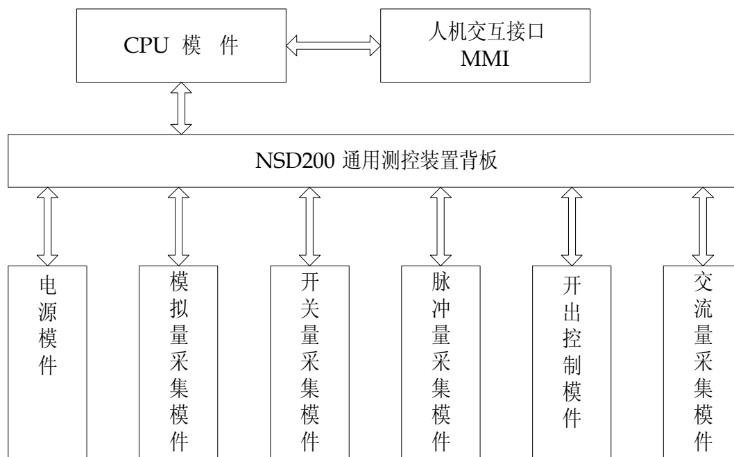
图 3.1 NSD200 系列通用测控装置原理框图
