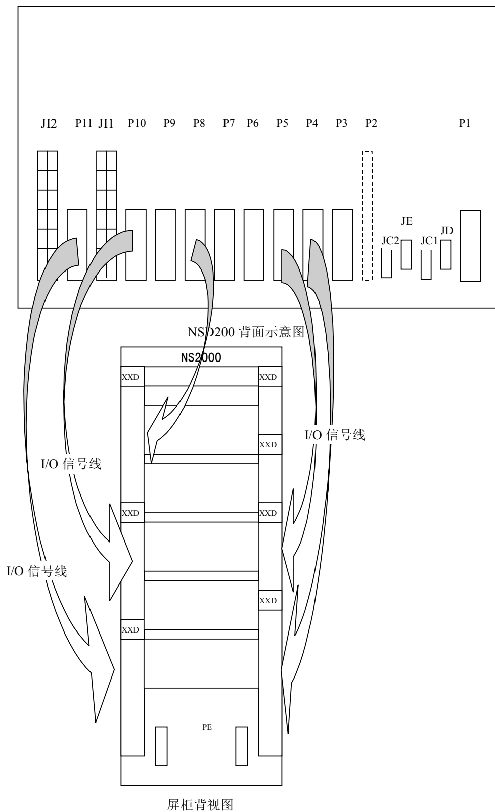
图 6.6 I/O 端子排接线图
