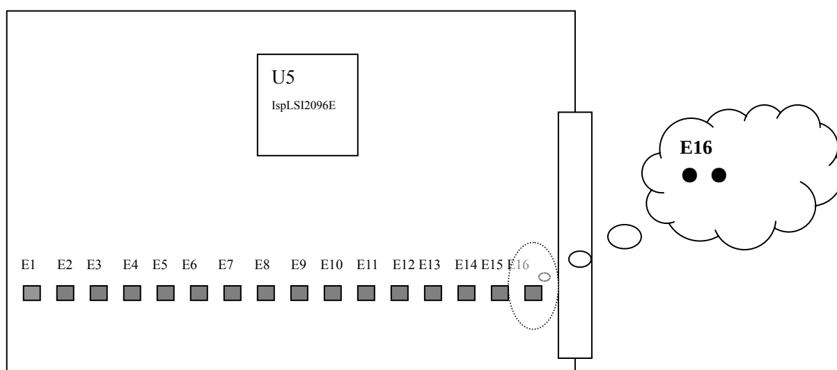
图 6.17 DI16A/PI16A 模件跳线位置图
