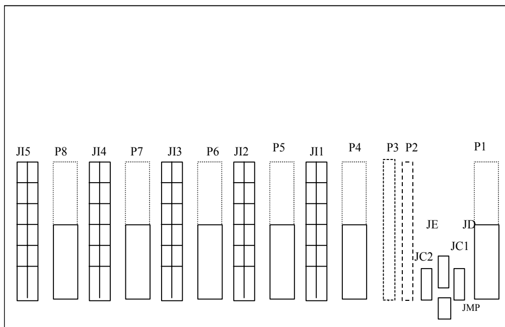
图 6.14 NSD203/NS206 背视图
