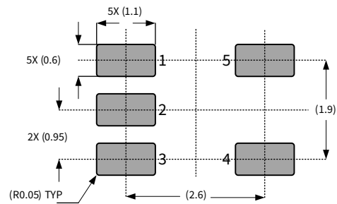
SOT23-5L
