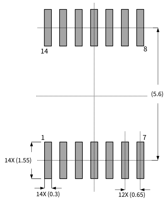
TSSOP14
