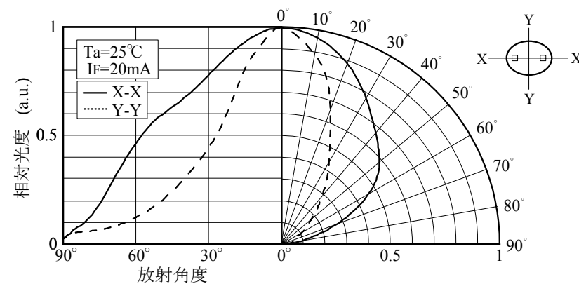
■ 指向特性（NSPB346BS）
