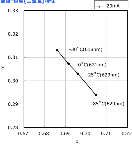
Ambient Temperature vs Chromaticity Coordinate ( \lambda_d ) 周囲温度-色度(主波長)特性
