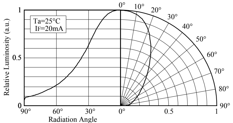
■ Directivity (NSPW515B(S))
