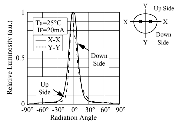
■ Directivity (NSPY800AS)
