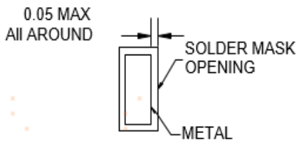
NON SOLDER MASK DEFINED
