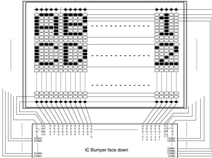
Type I (ADC=0, COM=1)
