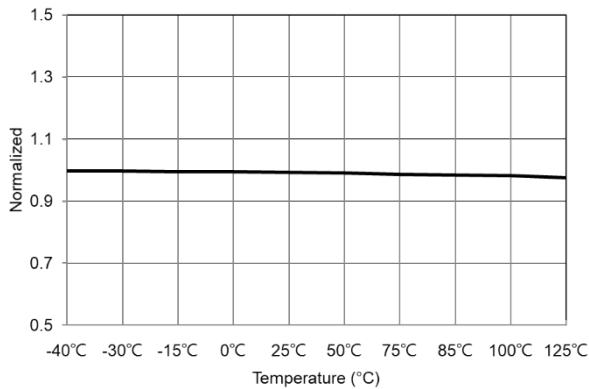
Fig. 11. Vcs_LIM_H
