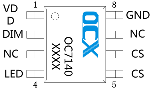
ESOP8
