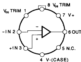
TO-99 (J-Suffix)
