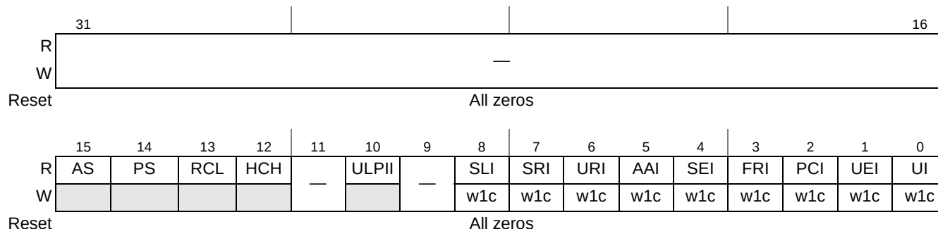
Figure 18-9. USB Status Register (USBSTS)
