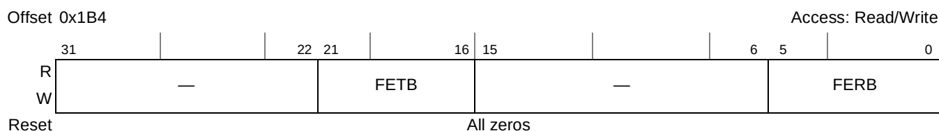
Figure 18-24. Endpoint Flush (ENDPTFLUSH)
