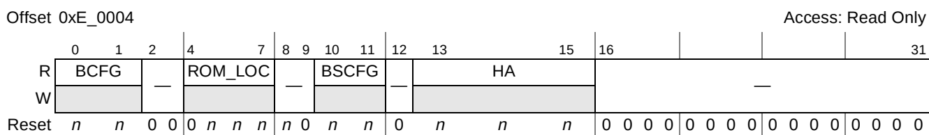
Figure 22-2. POR Boot Mode Status Register (PORBMSR)
