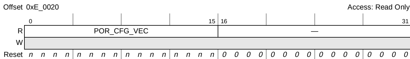
Figure 22-6. POR Configuration Register (GPPORCR)
