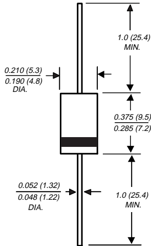
DO-201AD
