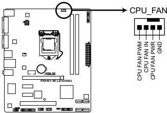
P8H61-M LE/USB3 CPU fan connector
